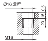
Çelik burçlu Referans Nr. 2520
