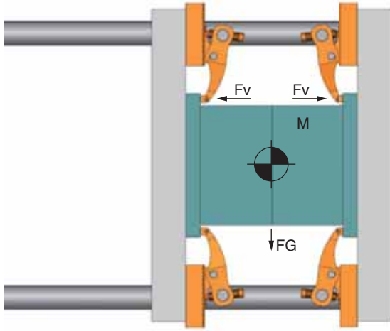
Enjeksiyon Kalıpları İçin Bağlama Şablonu Power Clamp For Injection Moulding
