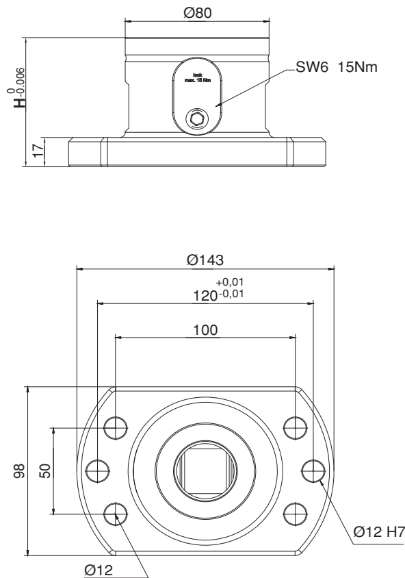
Ürün Nr. 0900 5-Eksen Blok Baęlama
