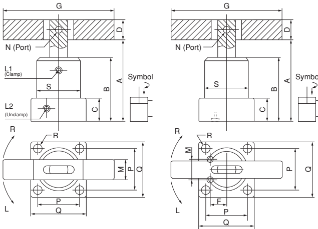
Ürün Nr. 1045 Hidrolik Dönmeli Bağlama Product Nr. 1045 Hydraulic Swing Clamp
