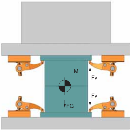
Pres Kalıpları İçin Bağlama Şablonu Power Clamp For Press Moulding
