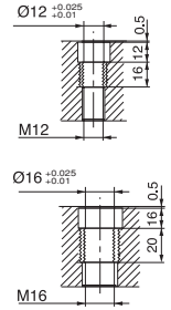
Çelik burçlu Referans Nr. 2540 Steel bush Reference No. 2540
